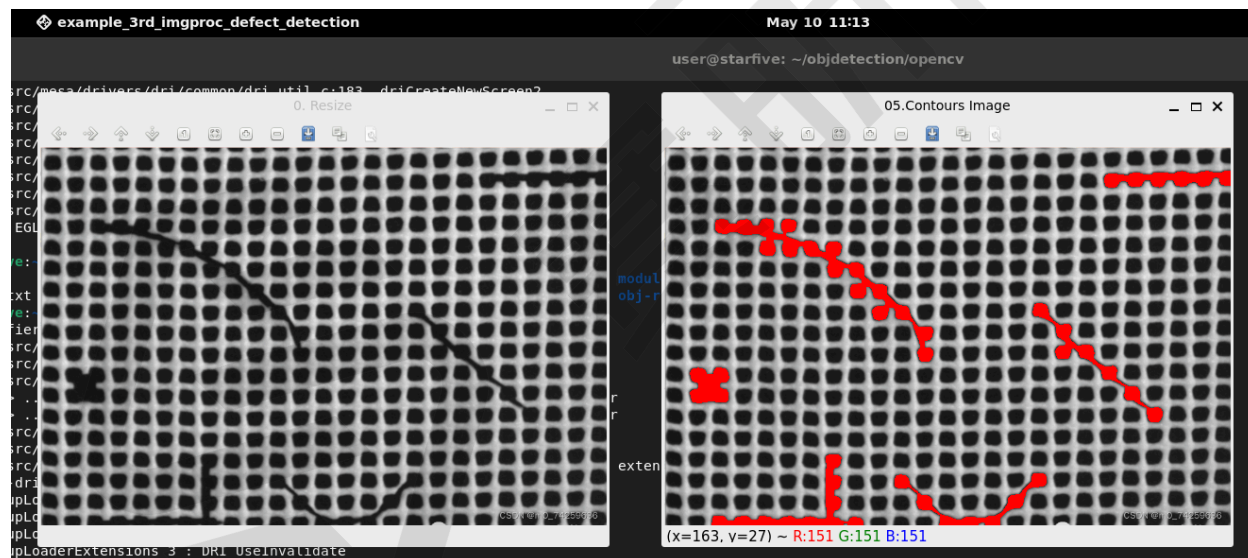
图 3-1 缺陷检测产品原图（左）与检测结果图（右）
