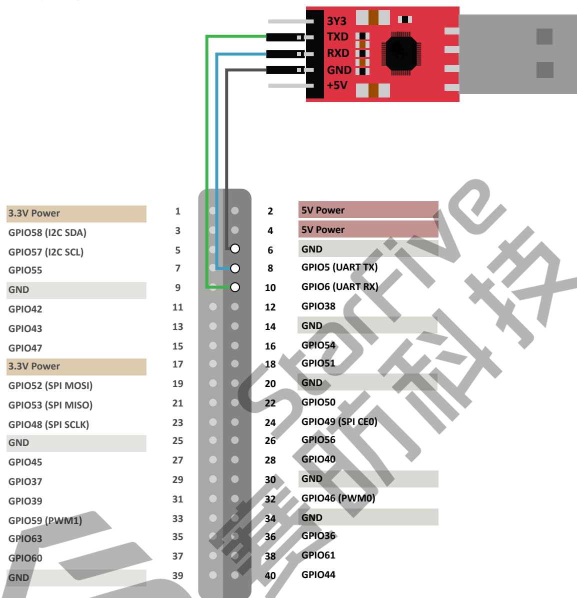
图 3-9 接跳线
