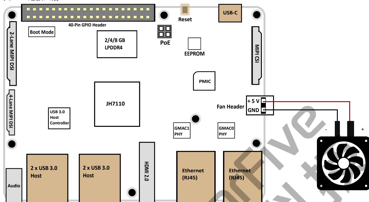
图 3-4 连接风扇
